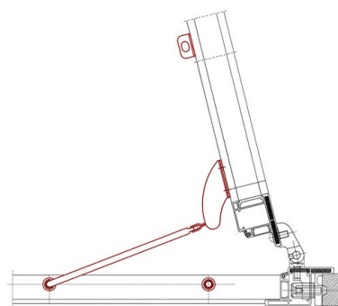
POSICIÓN INTERMEDIA
