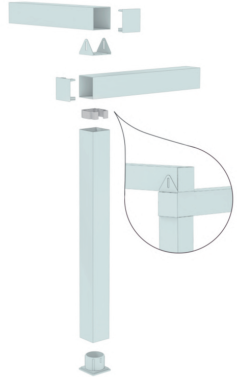
MONTAJE A DISTINTO NIVEL
