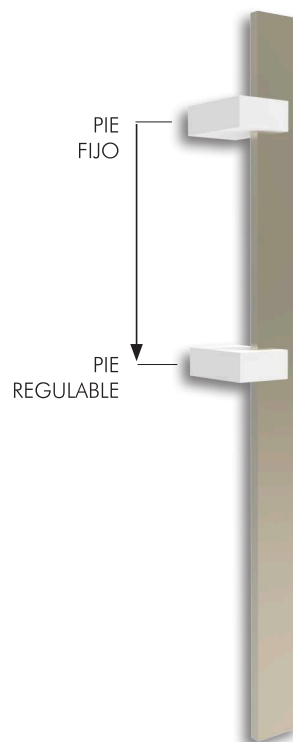
HORUS Largo 500 mm Pletina 40x8 mm Ref: THOR50- (simple) Ref: JTHOR50- (juego)
