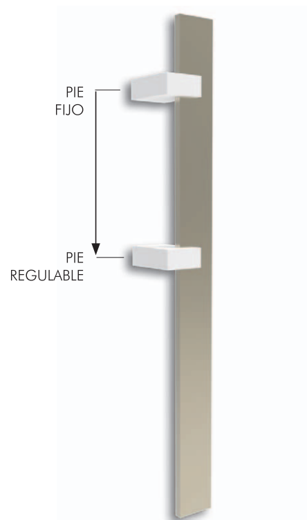
HORUS Largo 500 mm* Pletina 40x8 mm Ref: THOR50- (simple) Ref: JTHOR50- (juego)
